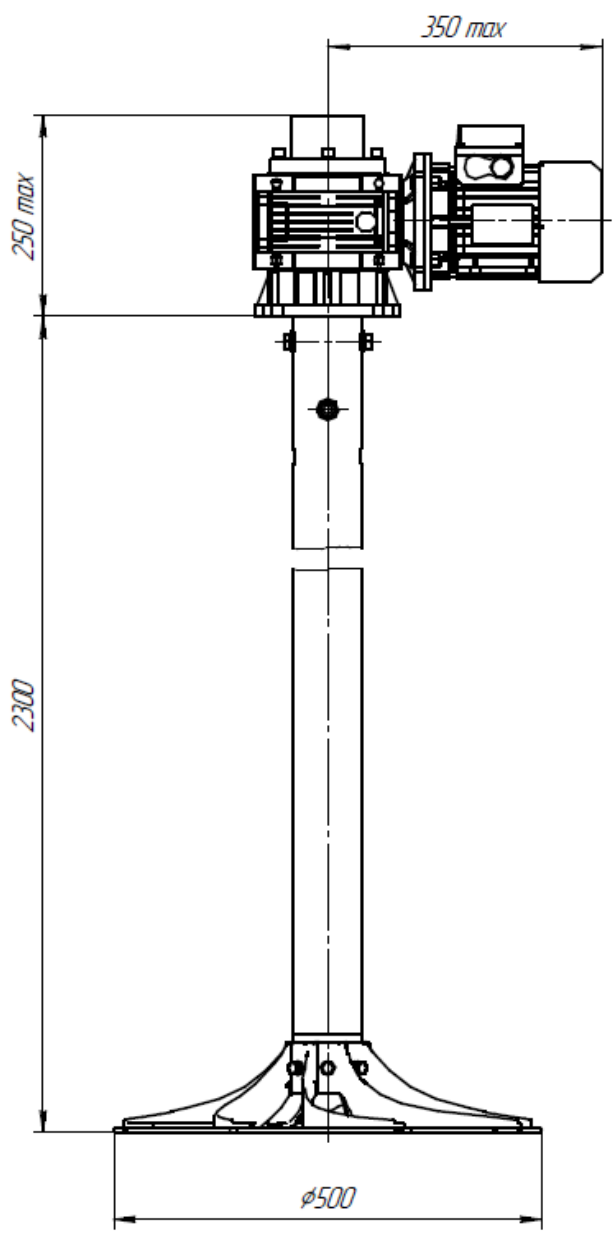
Габаритные размеры емкости ЦКТ 5000 с установленной мешалкой
