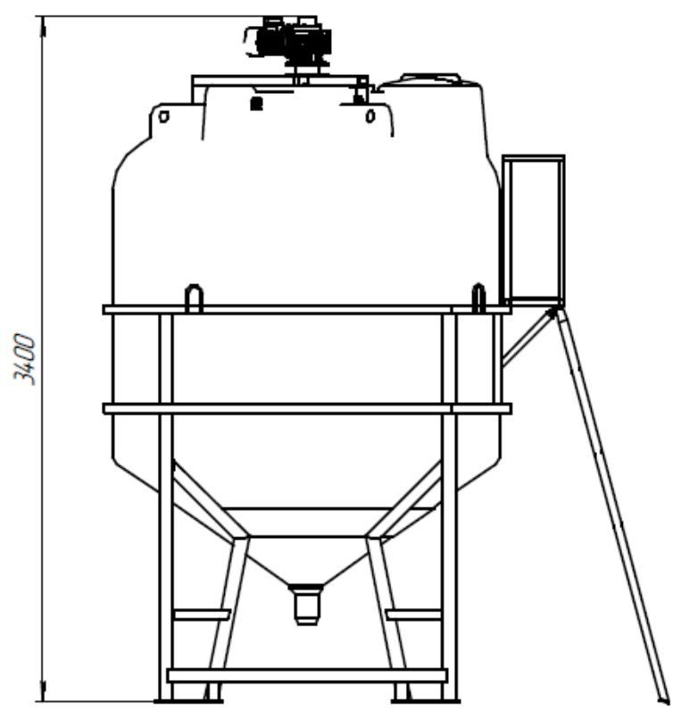
Габаритные размеры емкости ЦКТ 5000 с установленной мешалкой
